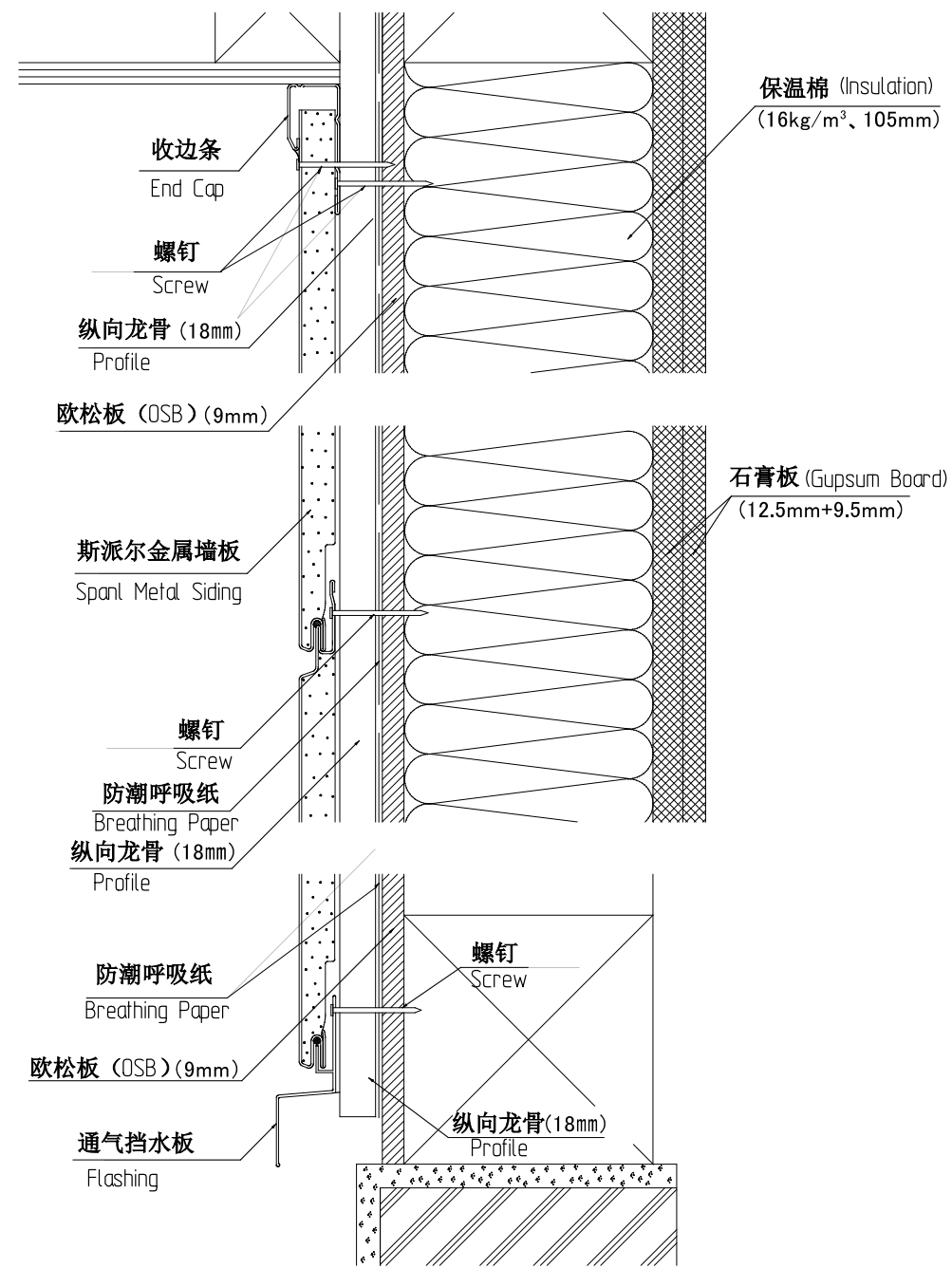
基本节点图 (纵向截面图) Section Drawing (Vertical View)
